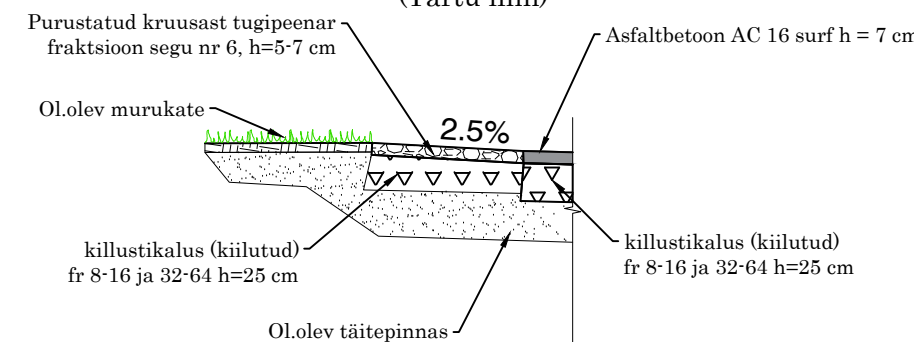
Tugipeenra ristlõige (Tartu linn)
