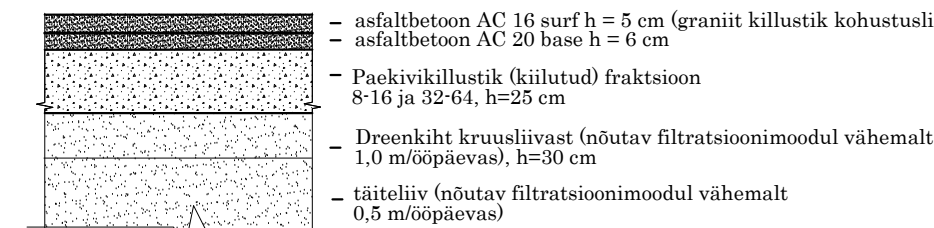
2. kihilise asfalkattega sõidutee kate taastamine
