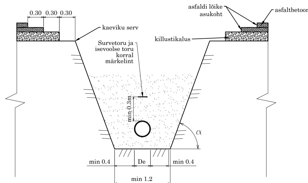
Kaeviku ristlõige 2 kihilise asfaldi korral Tüüp nr 2
