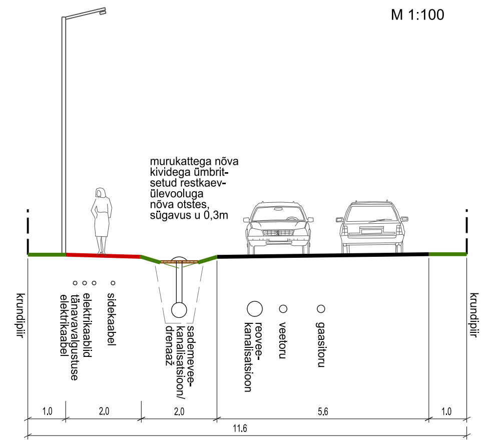
NÄITLIK TÄNAVA RISTLÕIGE A - A M 1:100
