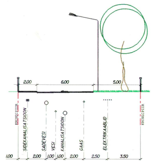
LÕIGE 2-2
