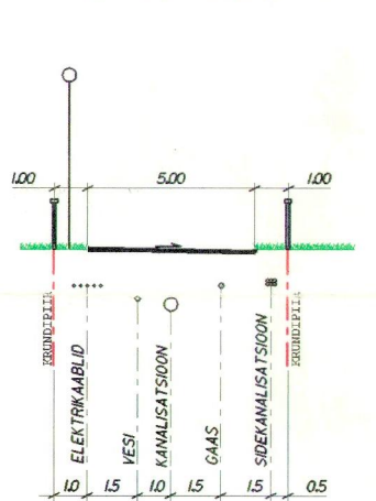
LÕIGE 3-3
