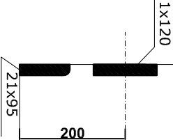
PÕRANDALISTUD M 1:10
