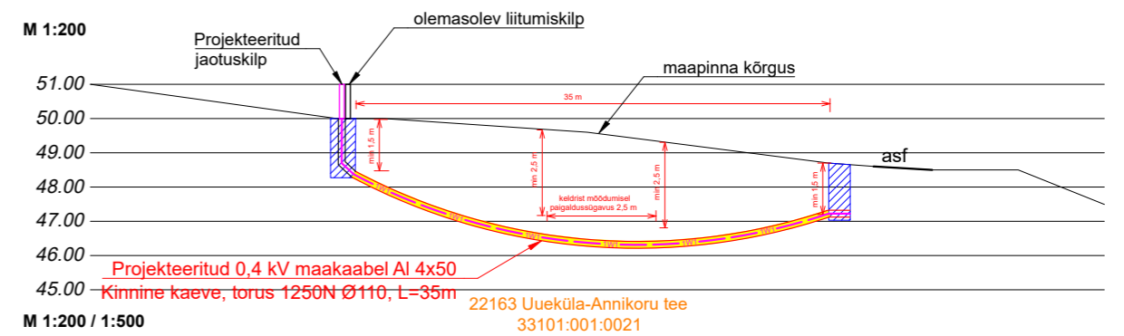
Kaabli pikiprofiili joonis 22163 Uueküla-Annikoru tee km 2,56 - 2,60 22163 Uueküla-Annikoru tee (33101:001:0021) maaüksusel
