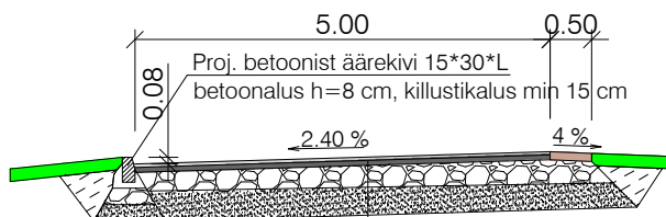
Lõige 2-2
