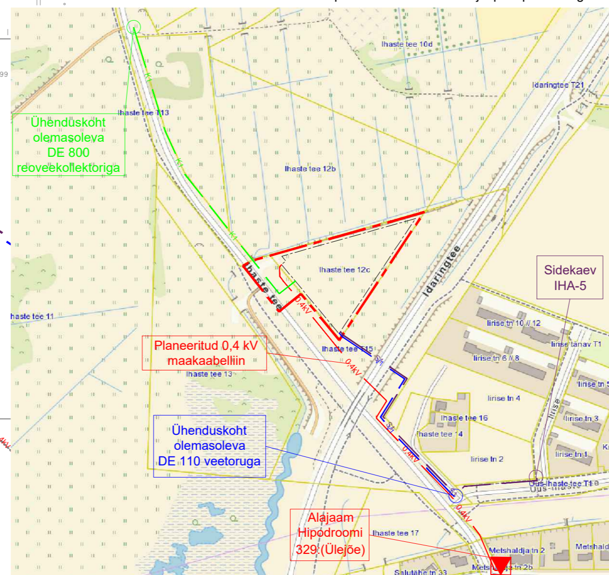
SKEEM 1. Planeeritud kanalisatsiooni-, vee-, elektri- ja sidetrasside põhimõtteline skeem väljaspool planeeringuala
