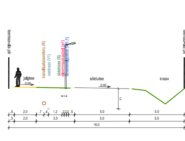
TEE LÕIGE 2-2 M 1 : 200
