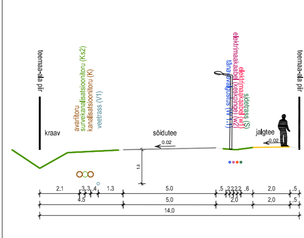
TEE LÕIGE 1-1 M 1 : 200
