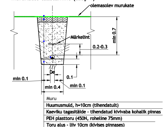
Kaeviku ristlõige. Tänavavalgustuskaabli paigaldus haljastala all. Murukatte taastamine (tüüp 4)
