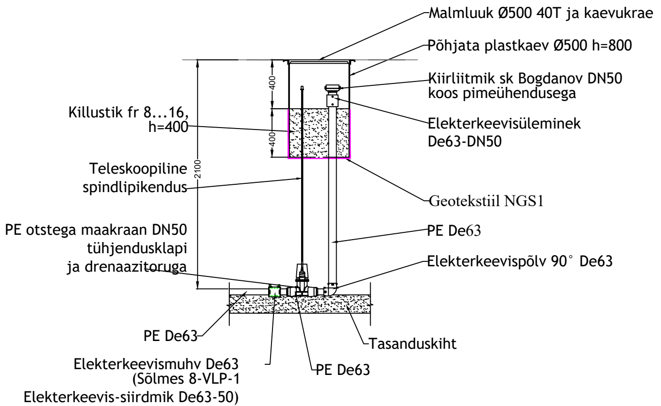
Lõige 1-1
