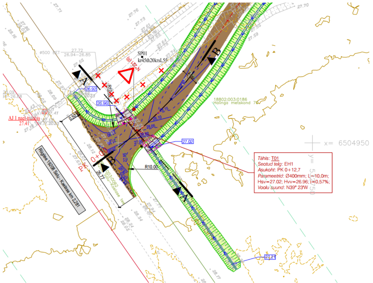
Joonis 1 Väljavõte ristumiskoha asendiplaani, vertikaalplaneerimise ja liikluskorralduse joonisest TL-4-11
