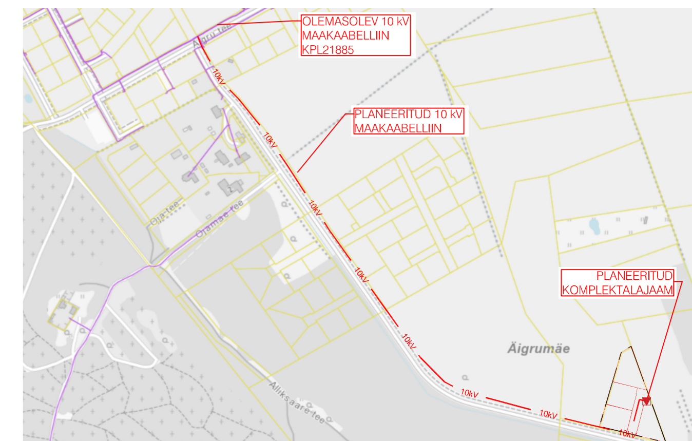
SKEEM 1. Planeeritud põhimõtteline elektrivarustuse skeem väljaspool planeeringuala
