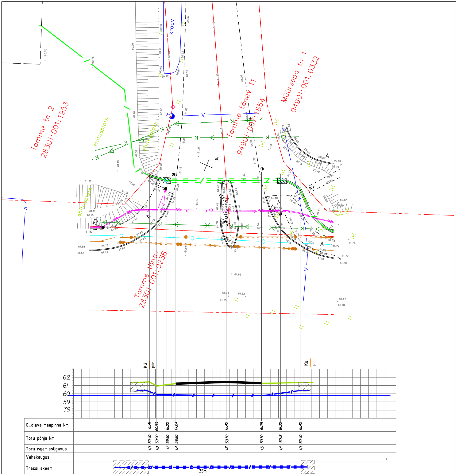
Ristumine 2 Tallinn-Tartu-Võru-Luhamaa tee T27 km. joonis 1
