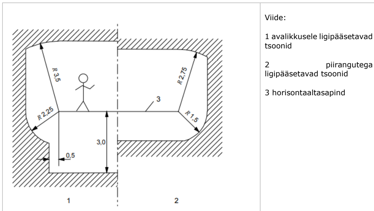
Joonis 4. Minimaalsed õhkvaheemikud sõiduki välisküljel asuvate pingestatud osade ja kontaktõhuliinisüsteemide pingestatud osade vahel, samuti inimeste poolt ligipääsetavate pingestatud osade vahel (EN 50122-1)
