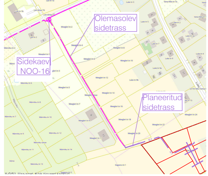
SKEEM 1. Sidevarustuse skeem väljaspool planeeringuala.
