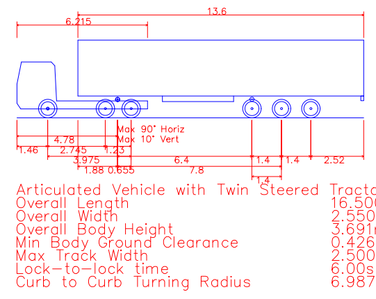
16,5 sadulrongi pöördekoridor (väline gabariit)
