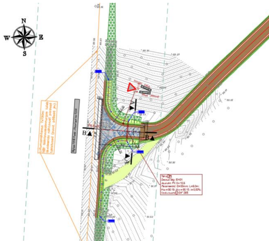
Joonis 1 Väljavõte ristumiskoha asendiplaani, vertikaalplaneerimise ja liikluskorralduse joonisest TL-4-11
