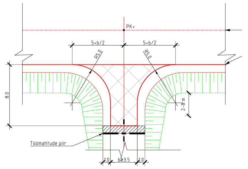
MAHASÕIDU TÜÜP I M 1 : 200
