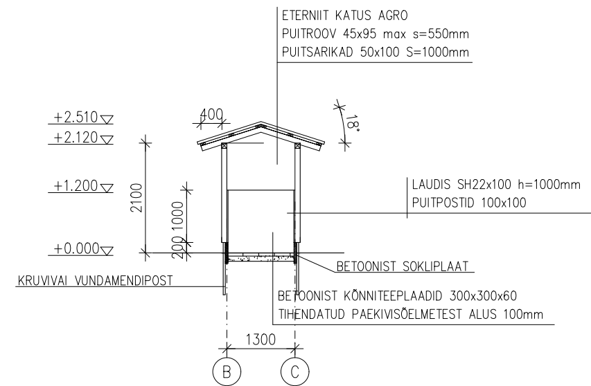
LÕIGE B-B 1:100
