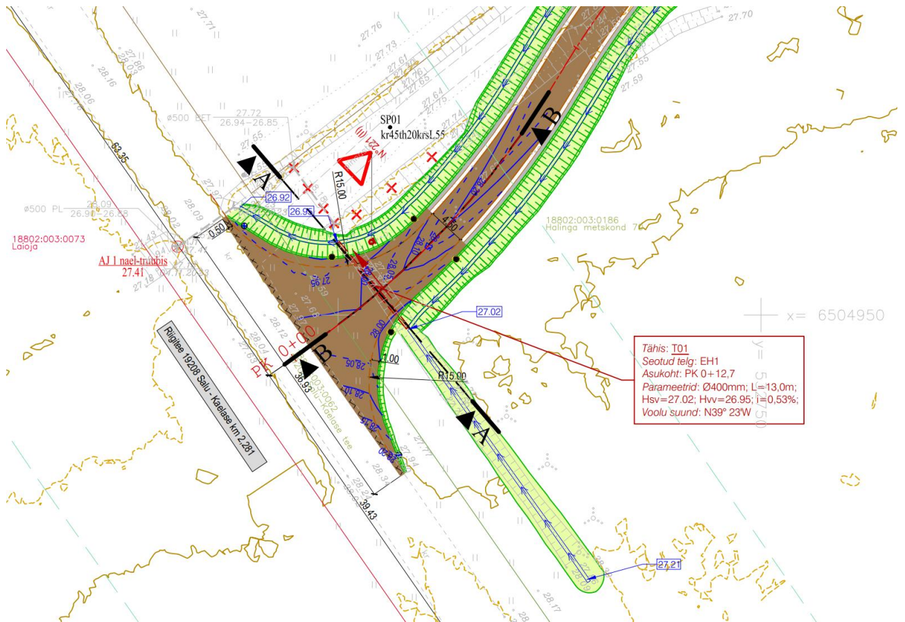
Joonis 1 Väljavõtte ristumiskoha asendiplaani, vertikaalplaneerimise ja liikluskorralduse joonisest TL-4-11
