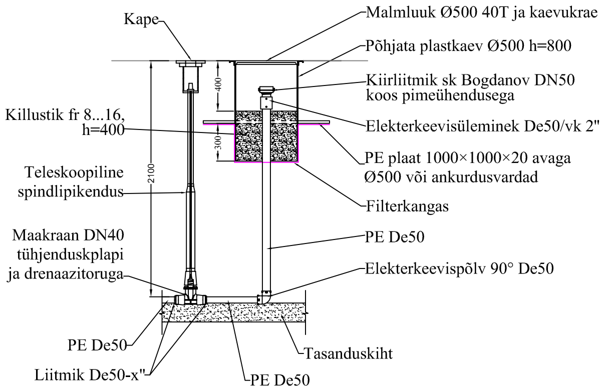
Lõige 1-1
