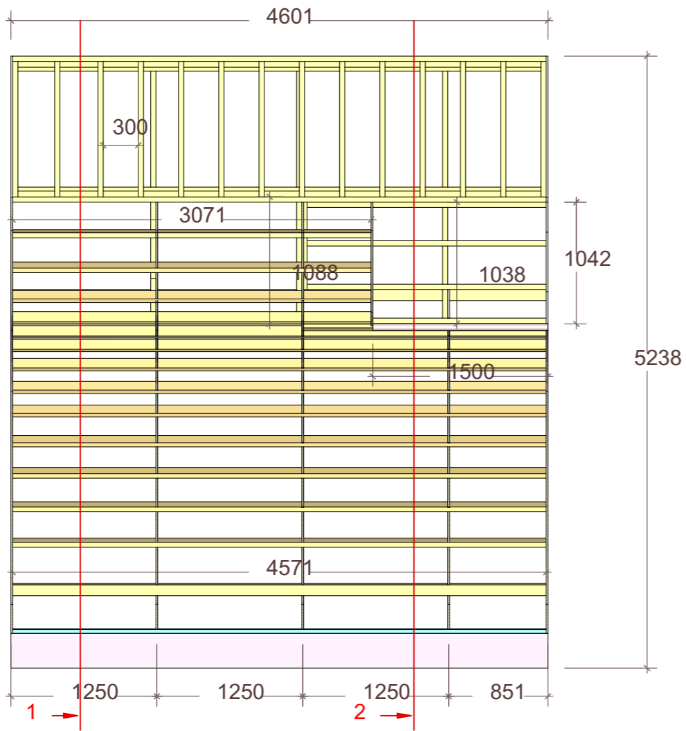
PEALTVAADE Mõõtkava 1:45
