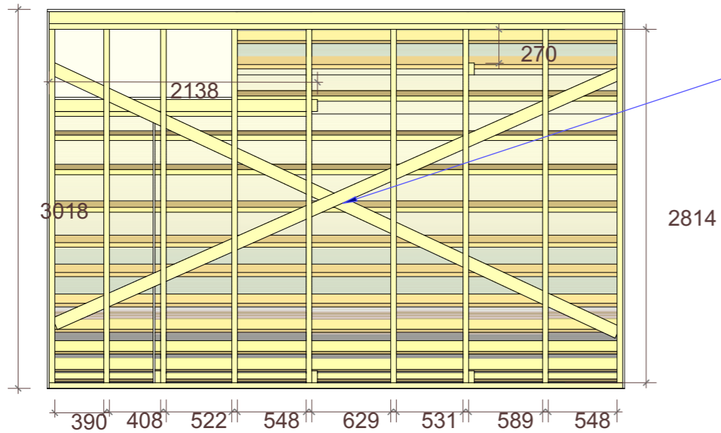
TAGANTVAADE Mõõtkava 1:45
