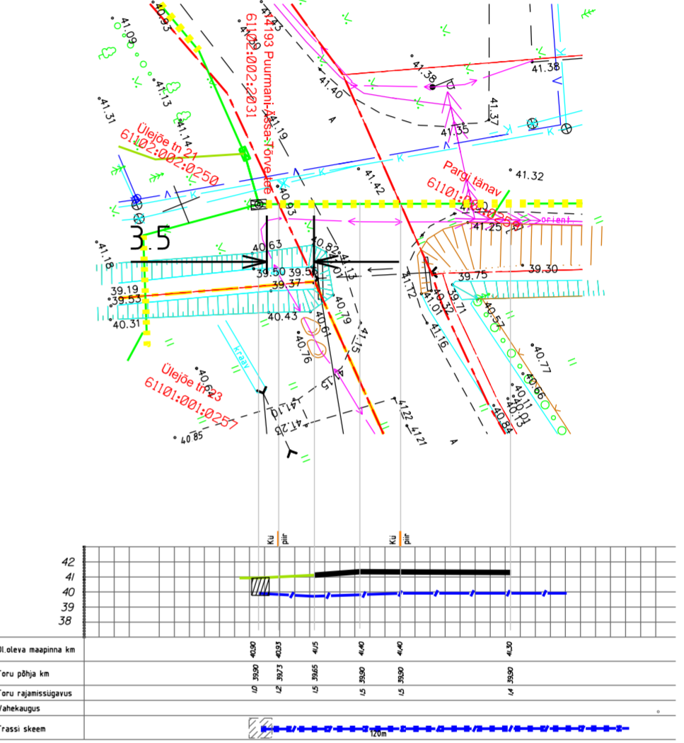
Ristumine 14193 Puurmani-Ässa-Tõrve tee km 0,81. joonis 8
