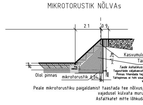
Ristumine 14193 Puurmani-Ässa-Tõrve tee km 0,14. joonis 6
