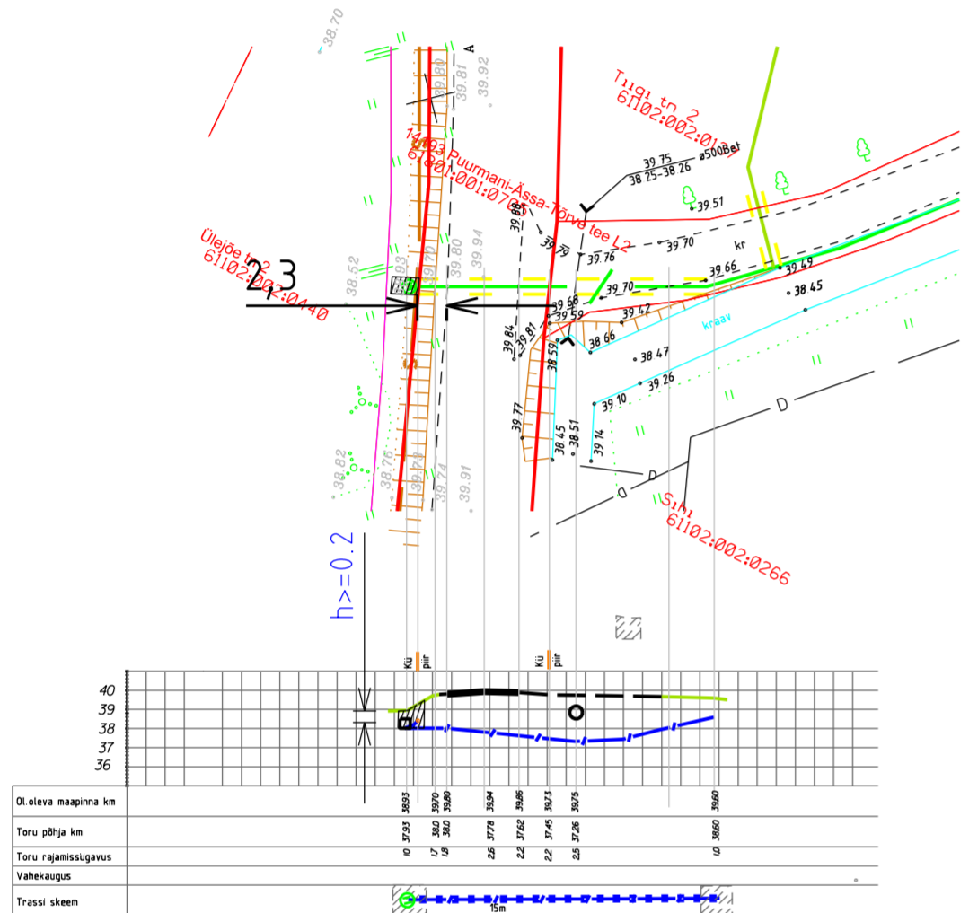
Ristumine 14193 Puurmani-Ässa-Tõrve tee km 0,14. joonis 6
