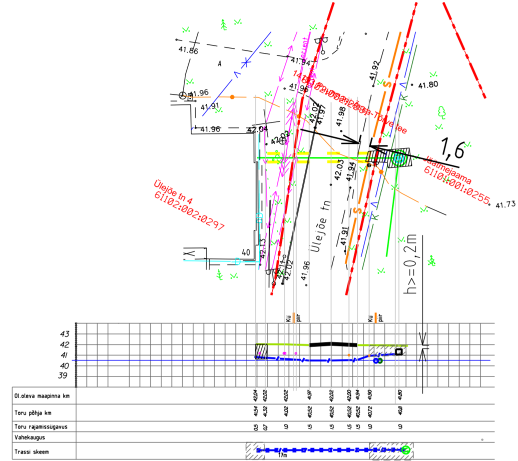
Ristumine 14193 Puurmani-Ässa-Tõrve tee km 0,41. joonis 7
