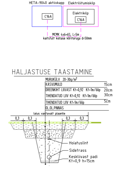
Elektritoitekaabli paigaldamise skeem
