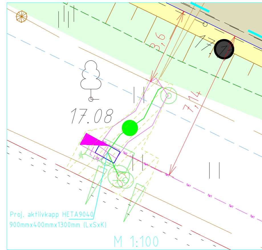
Elektritoitekaabli paigaldamise skeem
