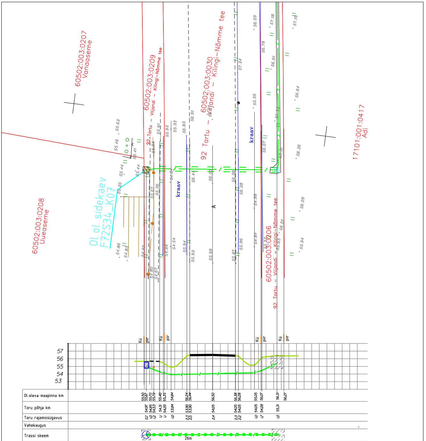
Ristumine 92 Tartu - Viljandi - Kilingi-Nõmme tee km 16.84. joonis 3
