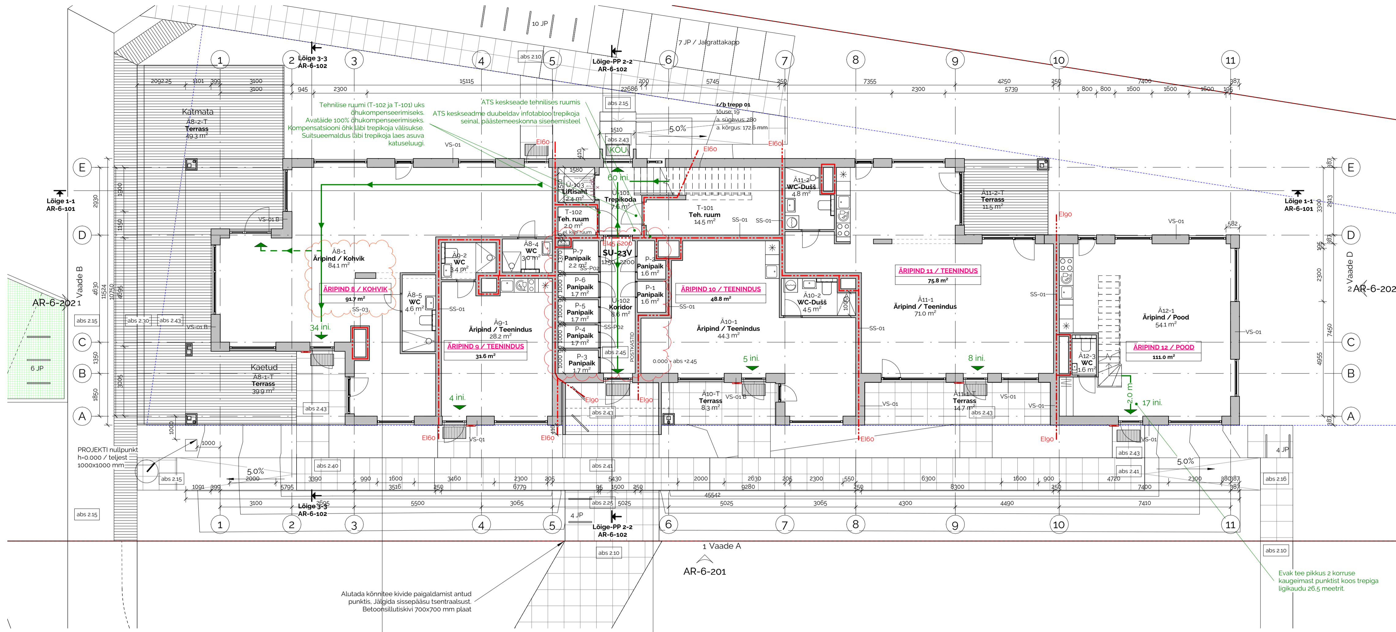
1 Korrus plaan 1:100
