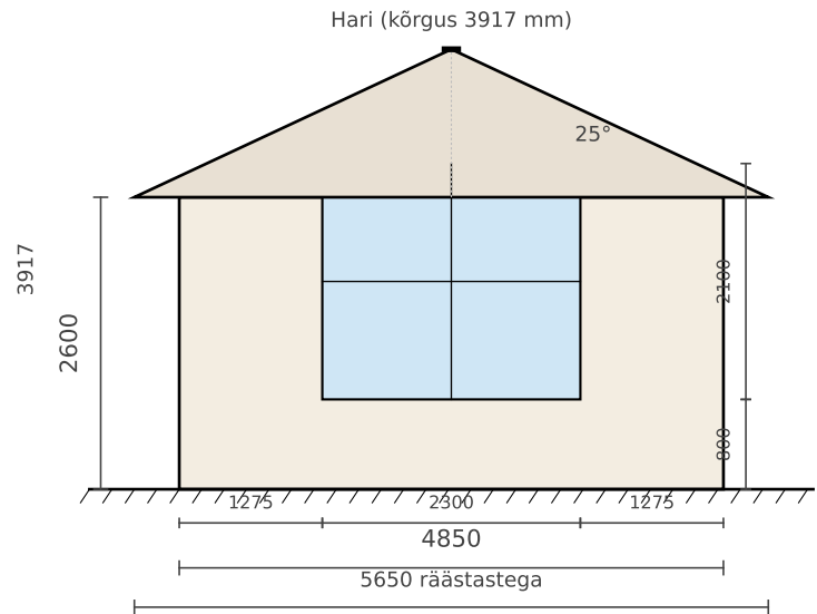
Parem külgvaade (idafassaad — räästaspool)
