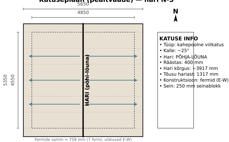
Katuseplaan (pealtvaade) — hari N-S
