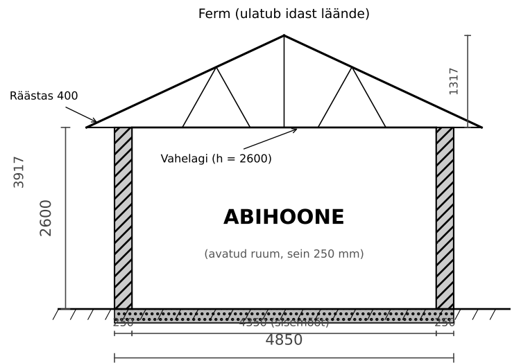
Lõige A-A (ida-lääne suunas, ristipidi harjaga)
