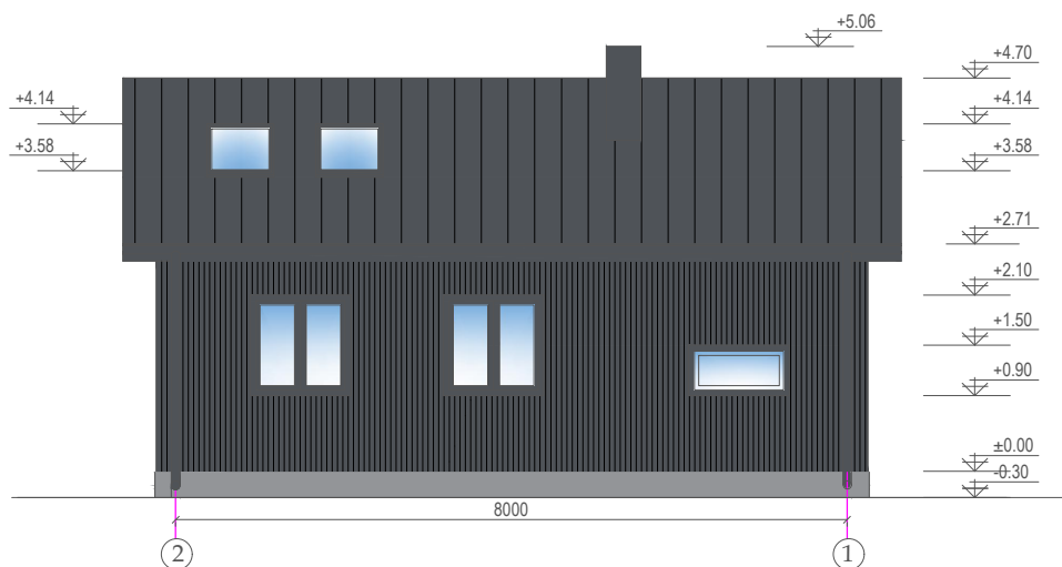
VAADE PÕHJAST M1:100
