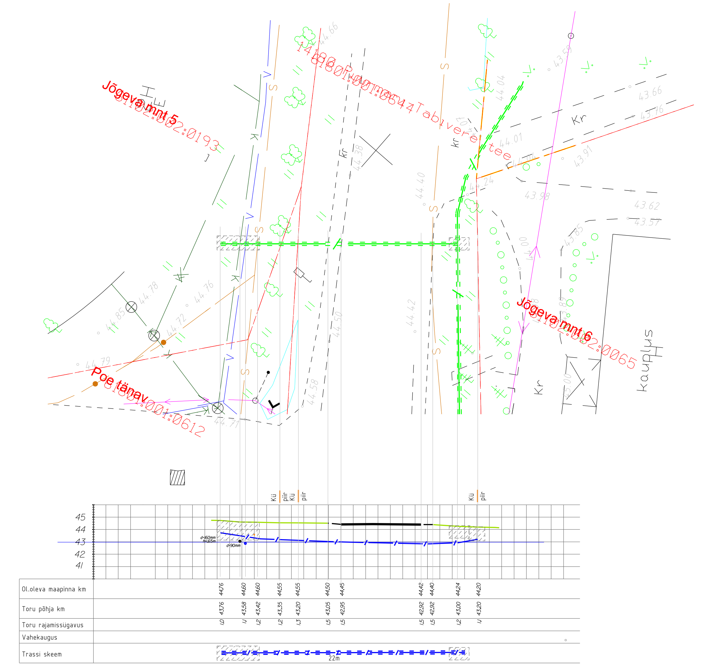
Ristumine 14180 Puurmani-Tabivere tee km 0,69. joonis 3
