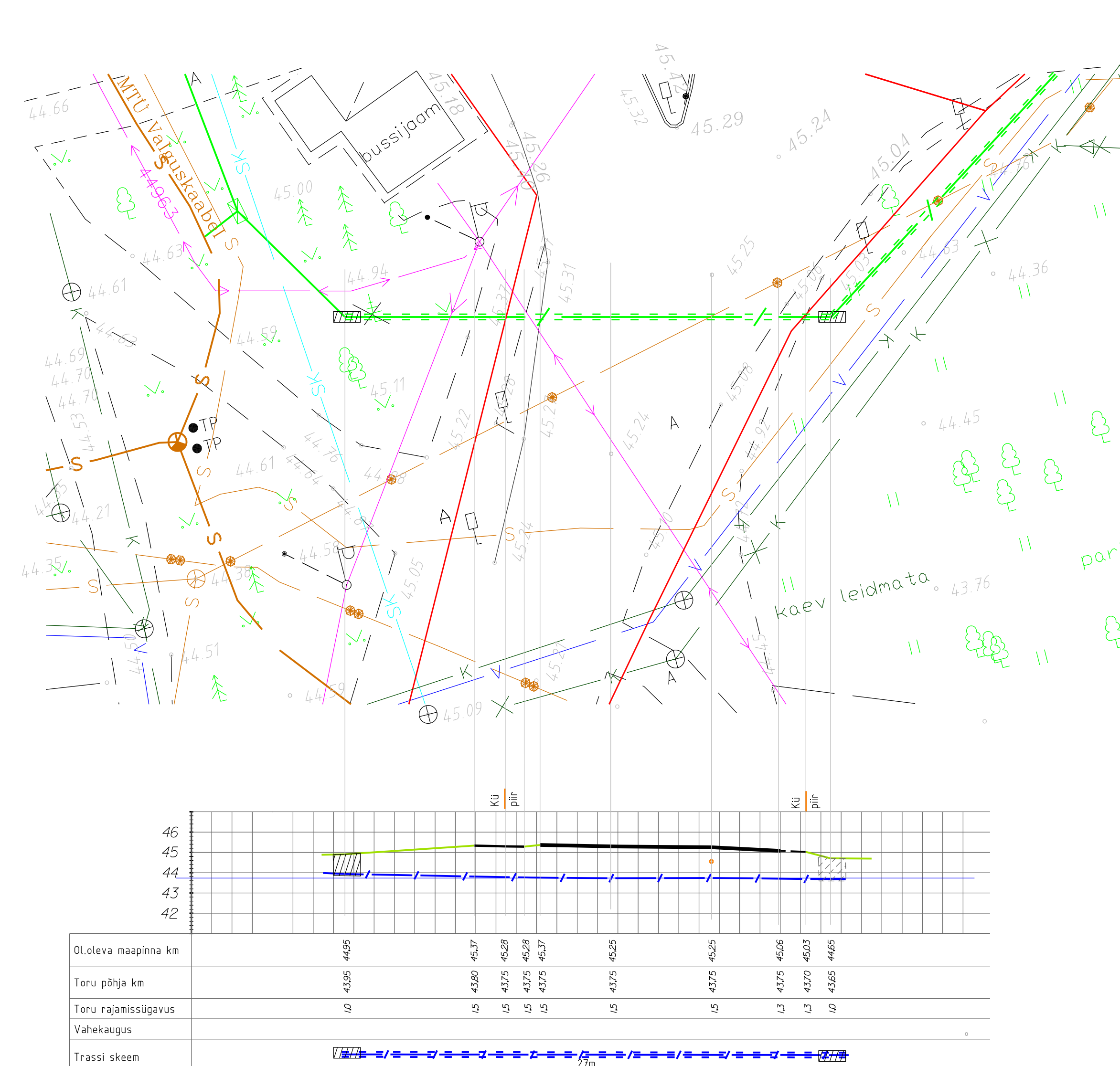
Ristumine 14180 Puurmani-Tabivere tee km 0,52 joonis 2
