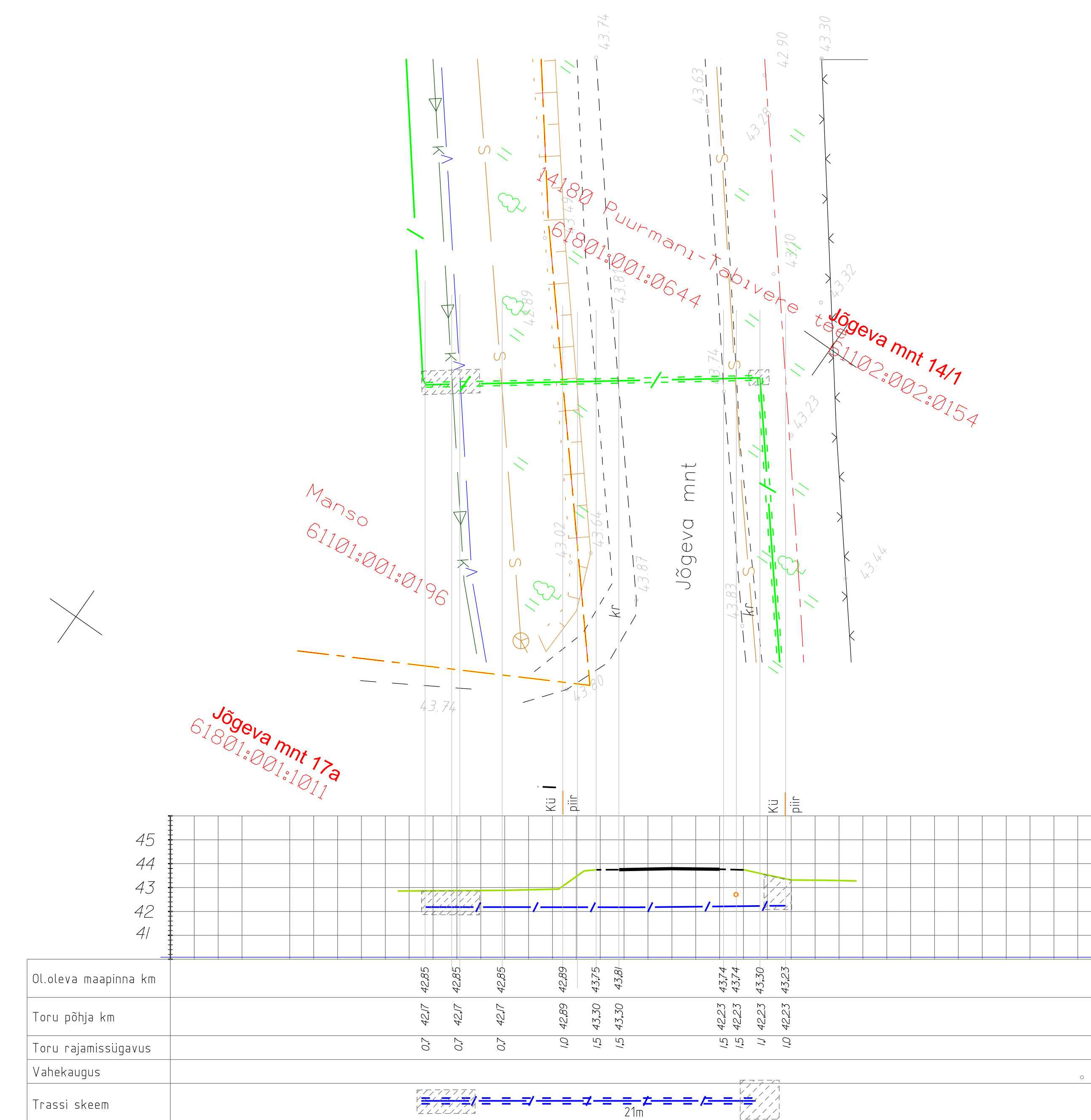
Ristumine 14180 Puurmani-Tabivere tee km 0,69. joonis 3
