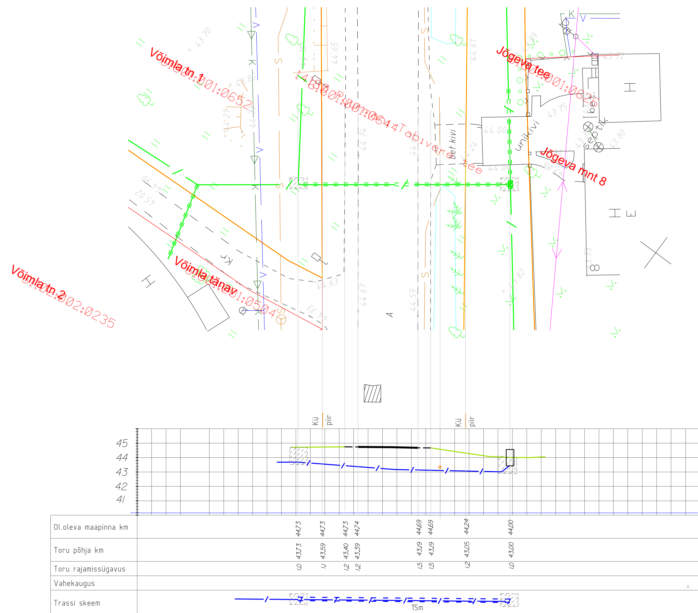
Ristumine 14180 Puurmani-Tabivere tee km 0,74. joonis 4
