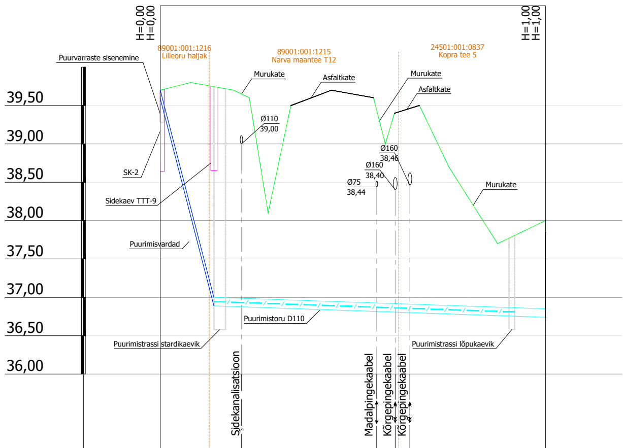
Puurimistrassi pikiprofiil
