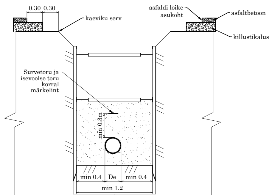
Kaeviku ristlõige Tüüp nr 2
