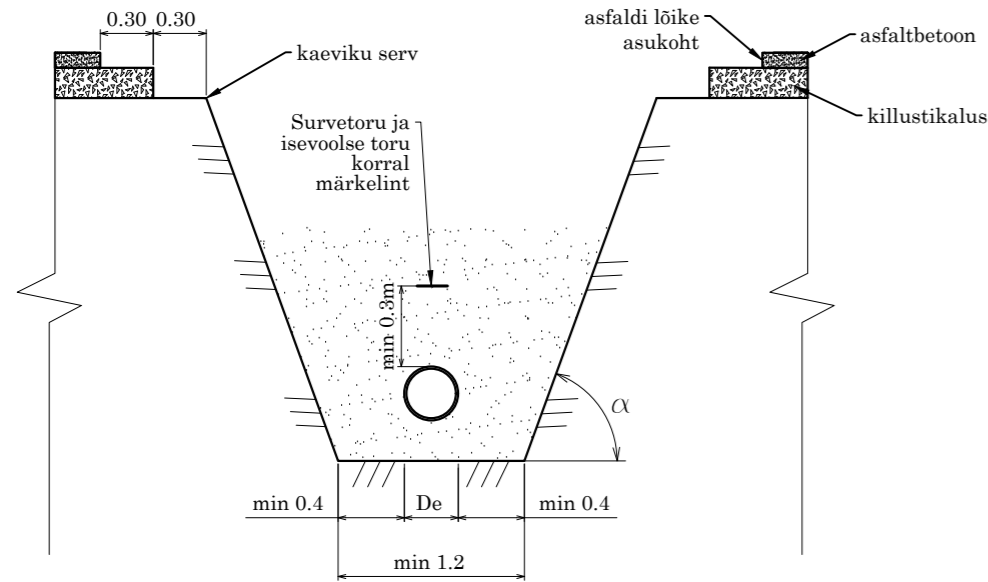
Kaeviku ristlõige Tüüp nr 1
