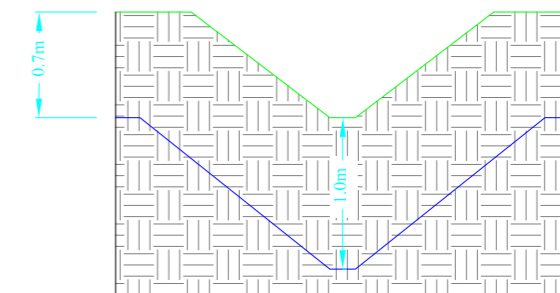
Projekteeritud mikrotoru
