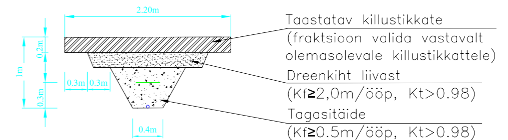
Kaeviku taastamine killustikkattega teel
