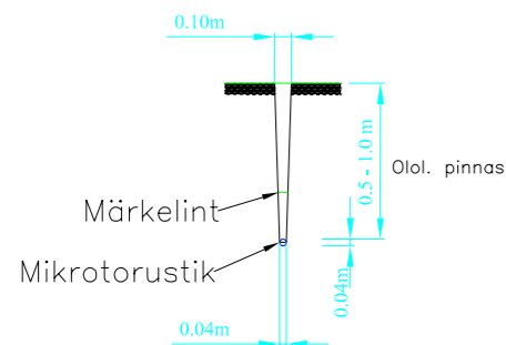
Kaevik paigaldusel kaabliadraga
