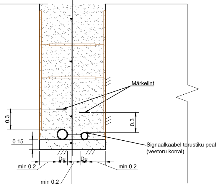
Toestatud kaeviku ristlõige (2 toru)
