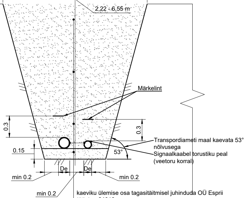
Kaeviku ristlõige (2 toru)
