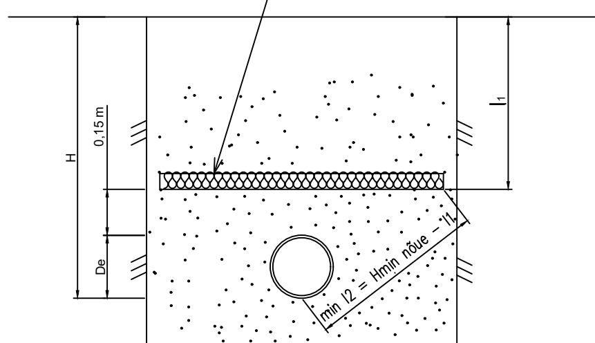
Soojustatud toru ristlõige soojustusplaat, h = 10\text{cm} ;
