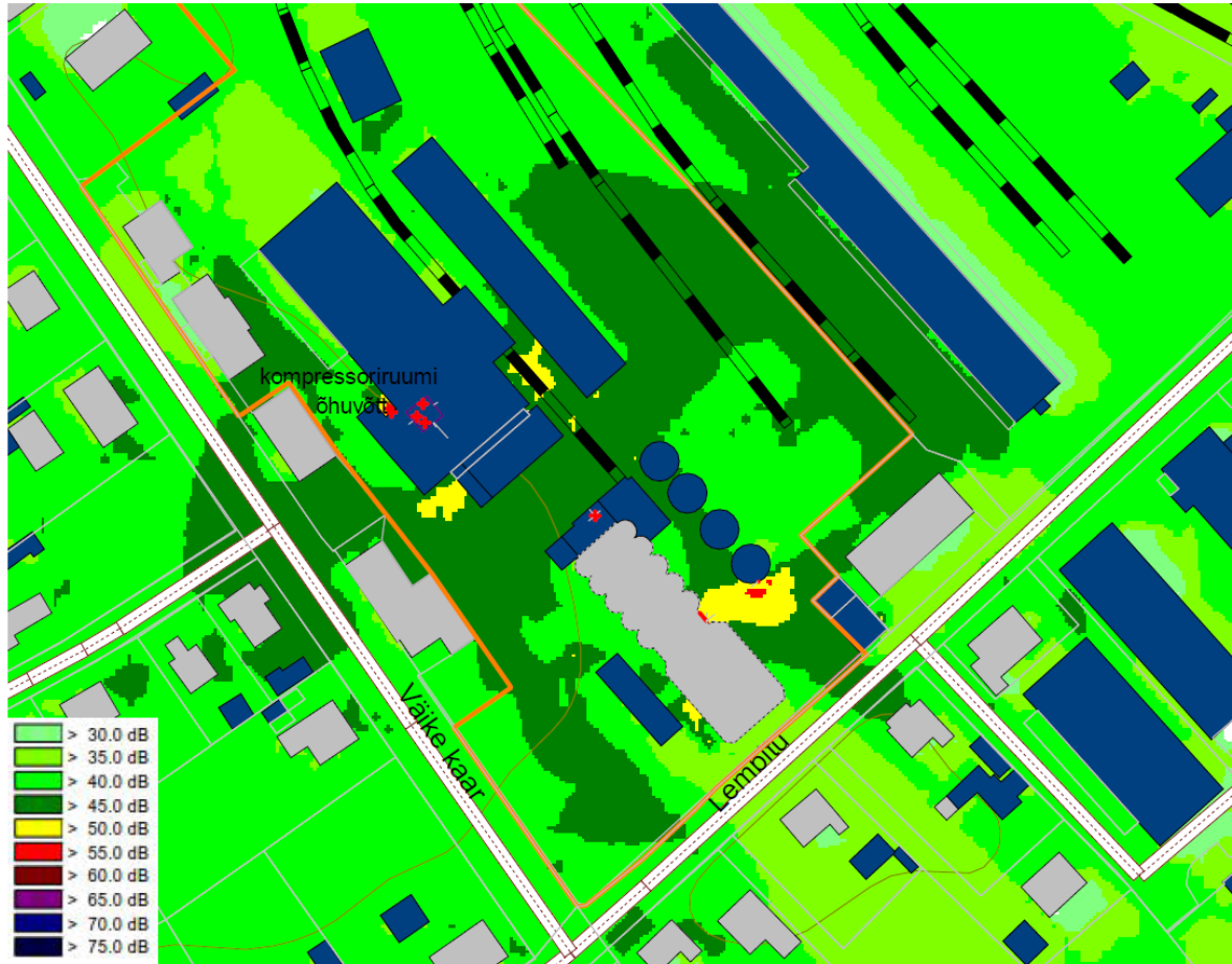
Joonis 14. Seadmete tööst tingitud hinnatud müratase päeval ajavahemikul leevendavate meetmete rakendamisel.
