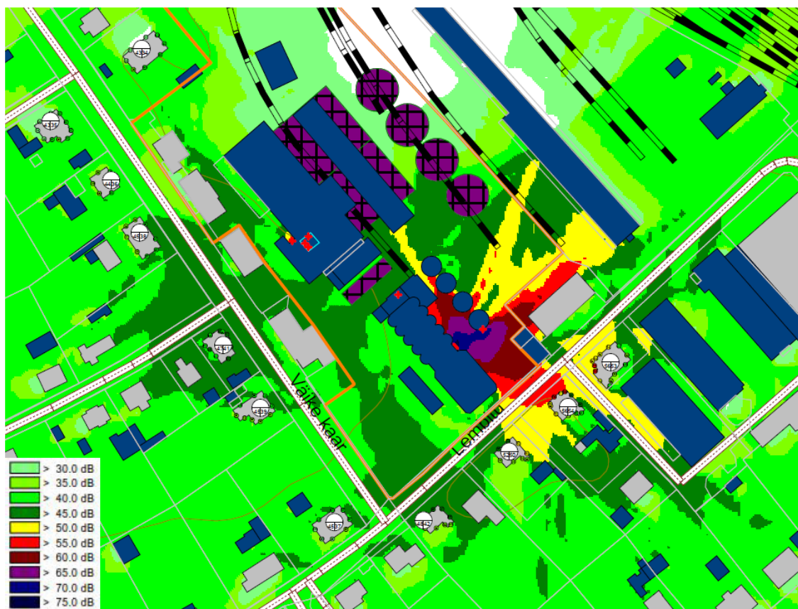
Joonis 11. Kõikide seadmete koos töötamisel esinevad hinnatud müratasemed päevasel ajavahemikul detailplaneeringu realiseerumisel. Ilma leevendavate meetmeteta.
