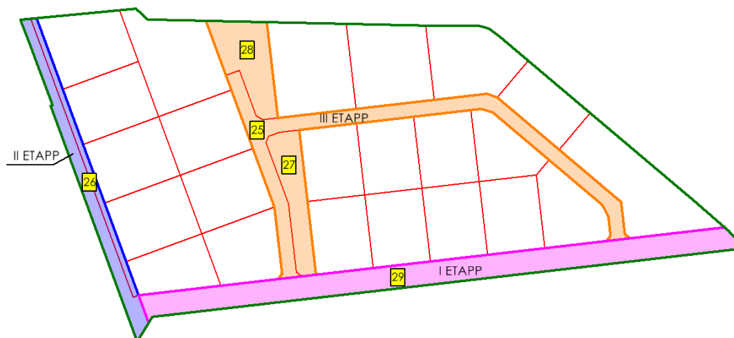
Skeem 4. Planeeringuala elluviimise etapid planeeritud tänava- ja üldkasutatava haljasala kruntide alusel. Planeeringuala on markeeritud rohelise joonega. Punase joonega on näidatud planeeritud krundipiirid. Roosa, sinise ja oranži tooniga on tähistatud vastavalt I, II ja III etapp.
