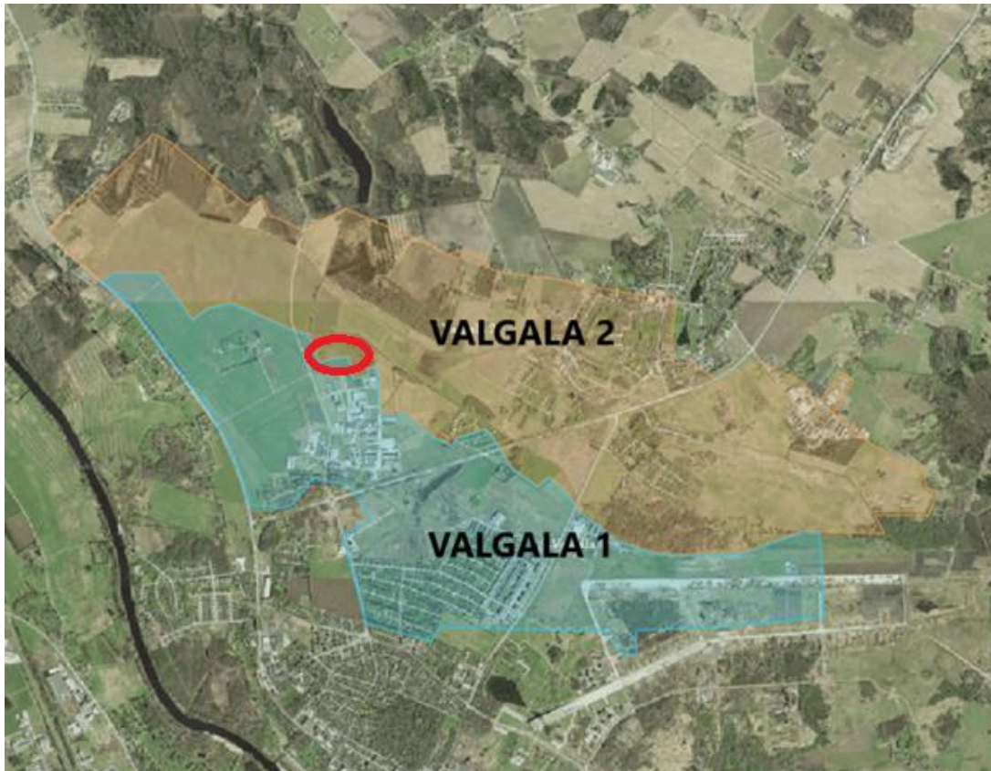
Skeem 3. Väljavõtte tööst „Tartu vald, Vahi, Raadi ja Kõrveküla aleviku ning Tila küla piirkonna sademevee kanalisatsiooni modelleerimine ja skeemi koostamine“ (Altren Projekt OÜ, töö nr 24067) valgalade kohta. Planeeringuala orienteeruv asukoht on tähistatud punase ovaaliga.
