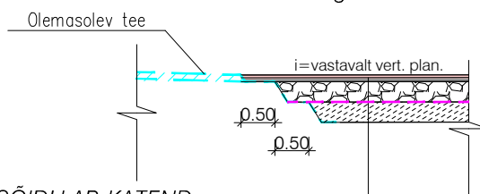
Lõige 1-1
