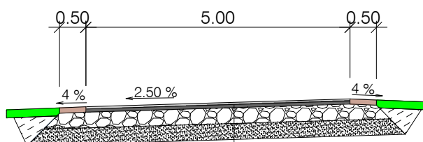
Lõige 2-2
