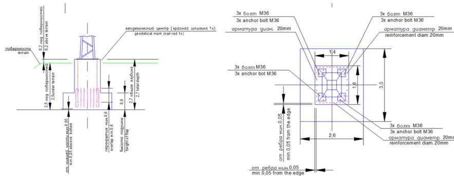
Joonis 5. Vundament HP100d
