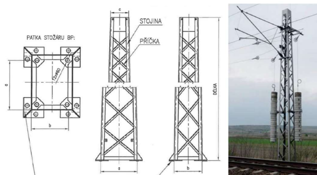
Joonis 7. BP-tüüpi mast
