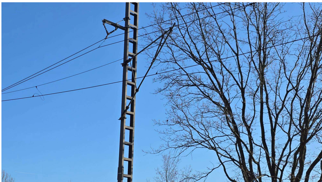
Foto 1: kontaktjuhtme tõstmine / kinnitamine tugifidrikonsoolile
