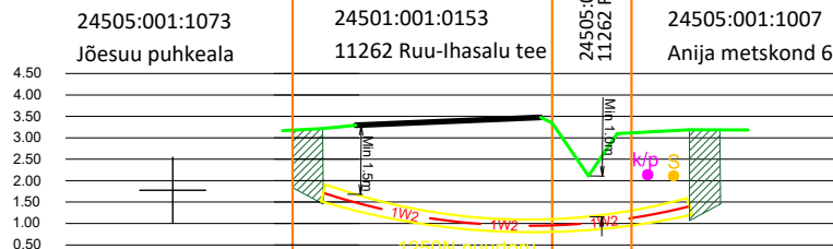
RISTMEVÄLJA JOONIS 1 Vahekaeviku puhul 11262 Ruu-Ihasalu tee Ristumine kinnisel meetodil km 5,84 L=21m
