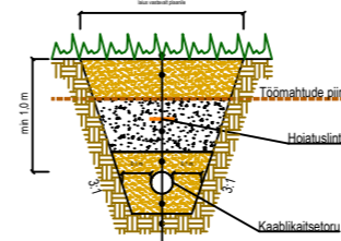
Kaablikaitseturu kaeviku lõige haljasala korral
