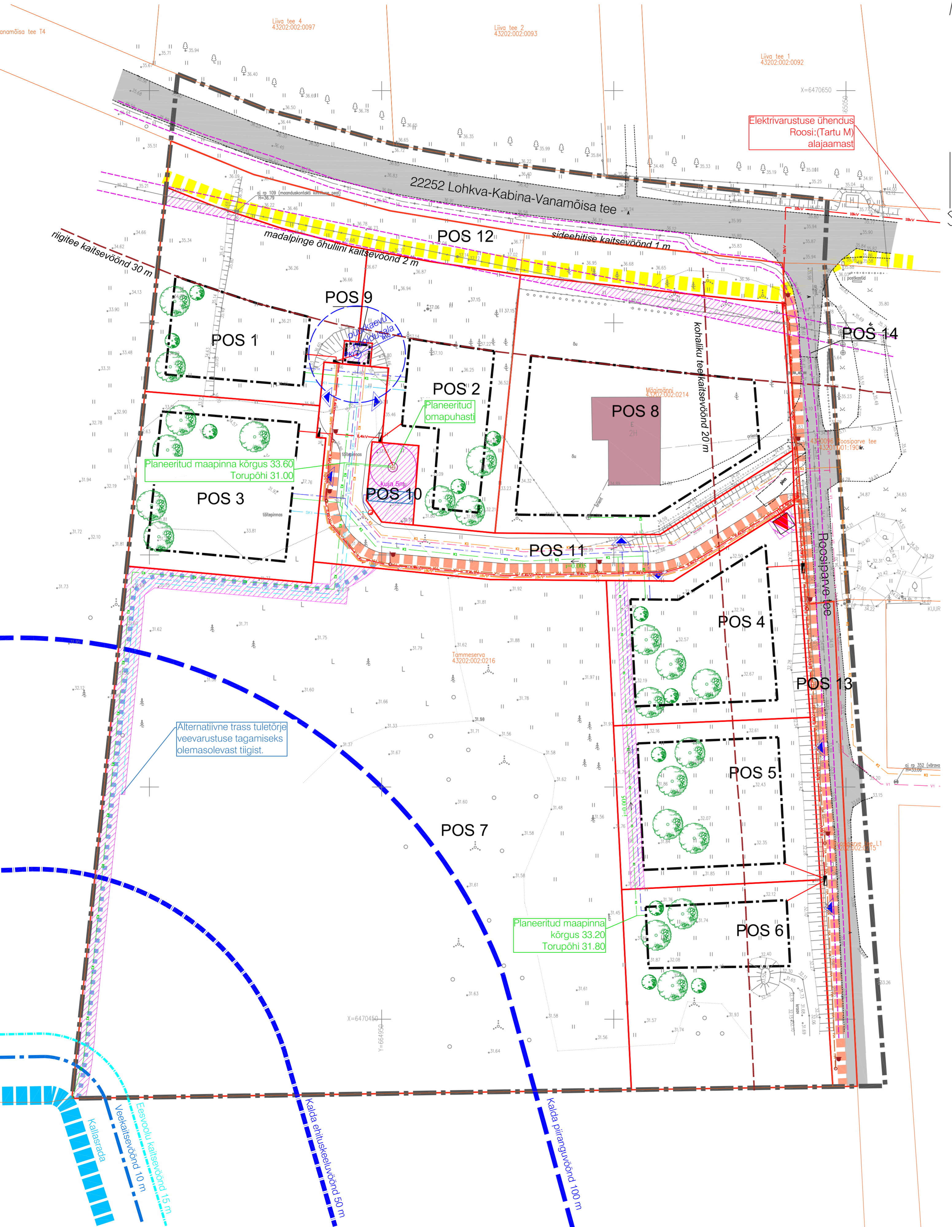
SKEEM 1. Planeeritud elektritoite põhimõtteline skeem väljaspool planeeringuala.
