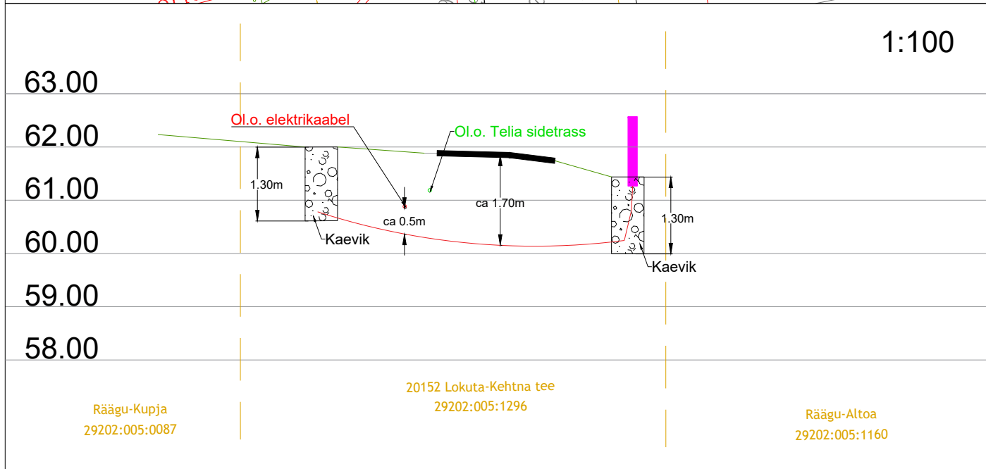
Ristumine 20152 Lokuta-Kehtna teega 12,65 km
