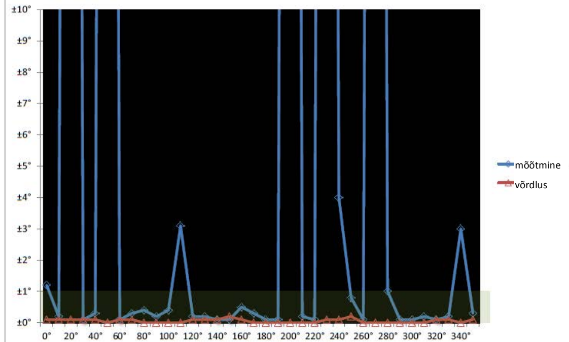
Peilingaator 4,6 kaugusel tuulepargist (MP 3) Direktsiooninurga näidu kõikumisvahemik, \lambda = 30 cm
