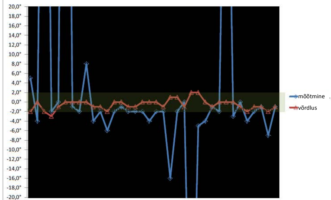
Peilingaator 4,6 kaugusel tuulepargist (MP 3) Kõrvalekalle regelikust suunast, \lambda = 30 cm
