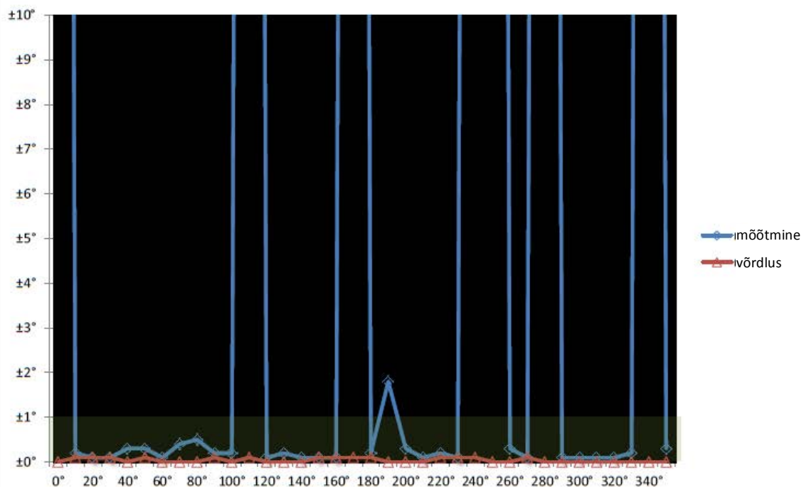
Peilingaator 4,6 kaugusel tuulepargist (MP 3) Direktsiooninurga näidu kõikumisvahemik, \lambda = 23 cm
