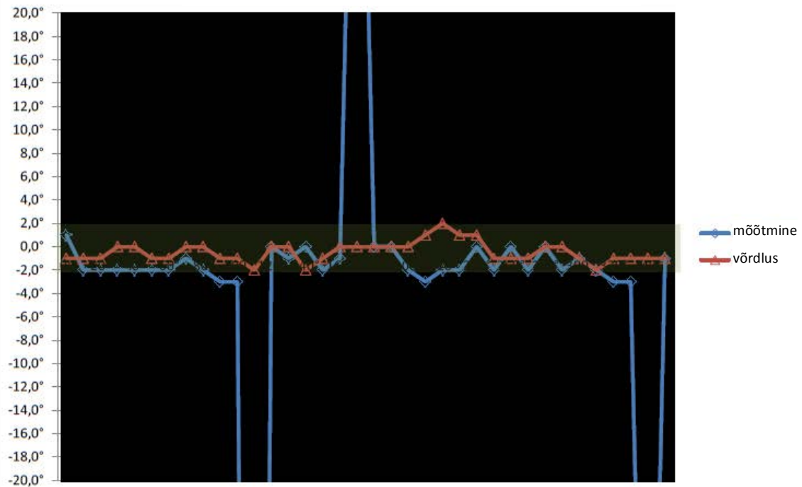
Peilingaator 4,6 kaugusel tuulepargist (MP 3) Kõrvalekalle regelikust suunast, \lambda = 23 cm
