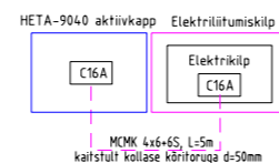
Elektritoitekaabli paigaldamise skeem
