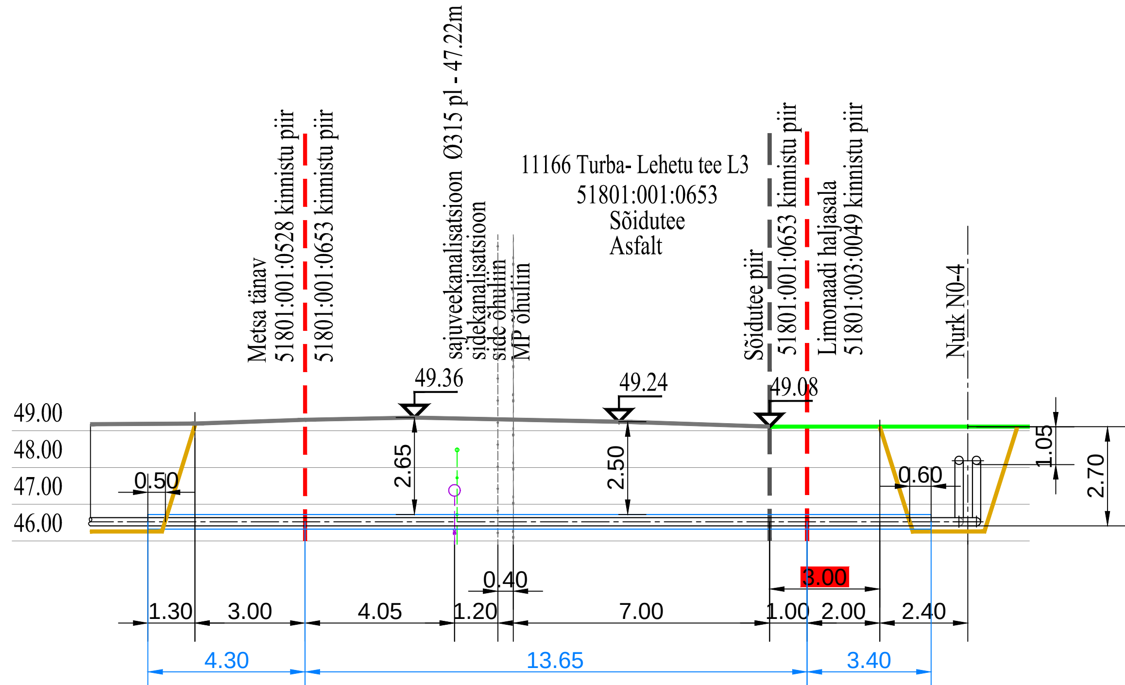
Lõige 2-2 M 1:100
