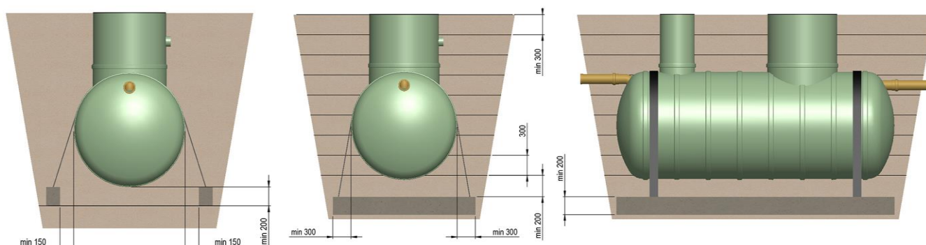
Biopuhasti ankurdamine
