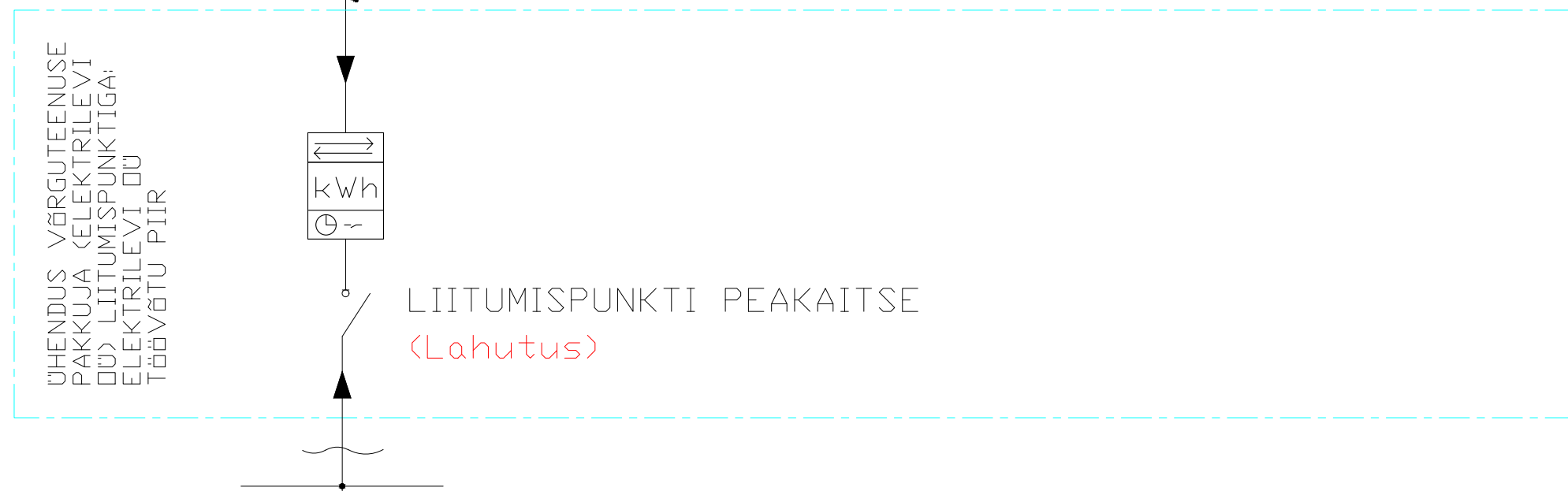
Põhimõtteline skeem ühe alajaama kohta
