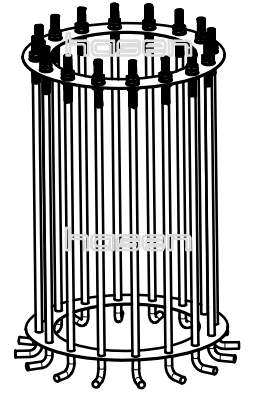
M33 X 16 Ankraj
