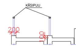
KOHTLÕIGE 4-4
