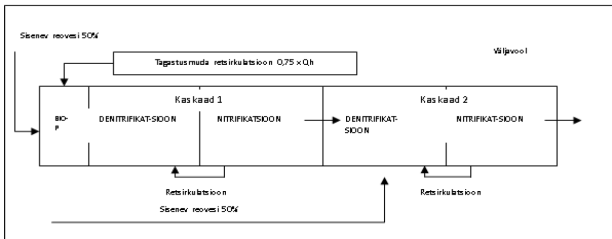
Joonis 6.2 Bioloogilise puhastuse põhimõtteline skeem
