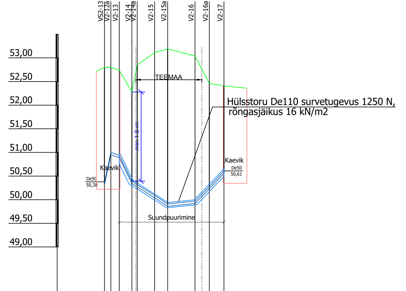
Pikiprofiil 2 13129 km 7.10
