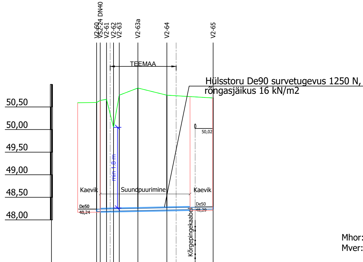
Pikiprofiil 1 13129 km 6.480
